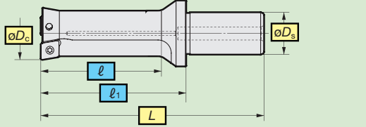
SEC-プランジドリルPDL型 SEC-Plunge Drill PDL Type
