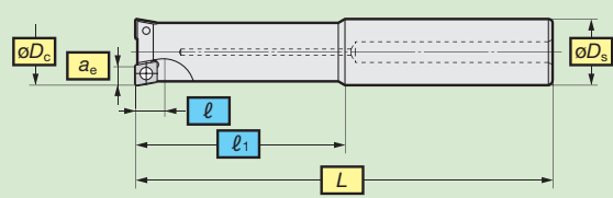
SEC-プランジミルPCT型 SEC-Plunge Mill PCT Type
